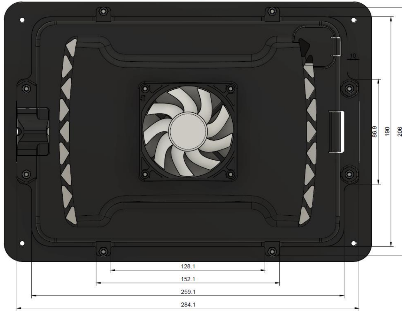
Platzbedarf hinter Panel SkyButler Pro 11" (iPad Pro 11" 1. - 3. Generation) Rückansicht
